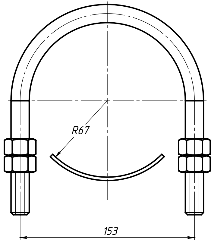
Поз.2 (Хомут)
